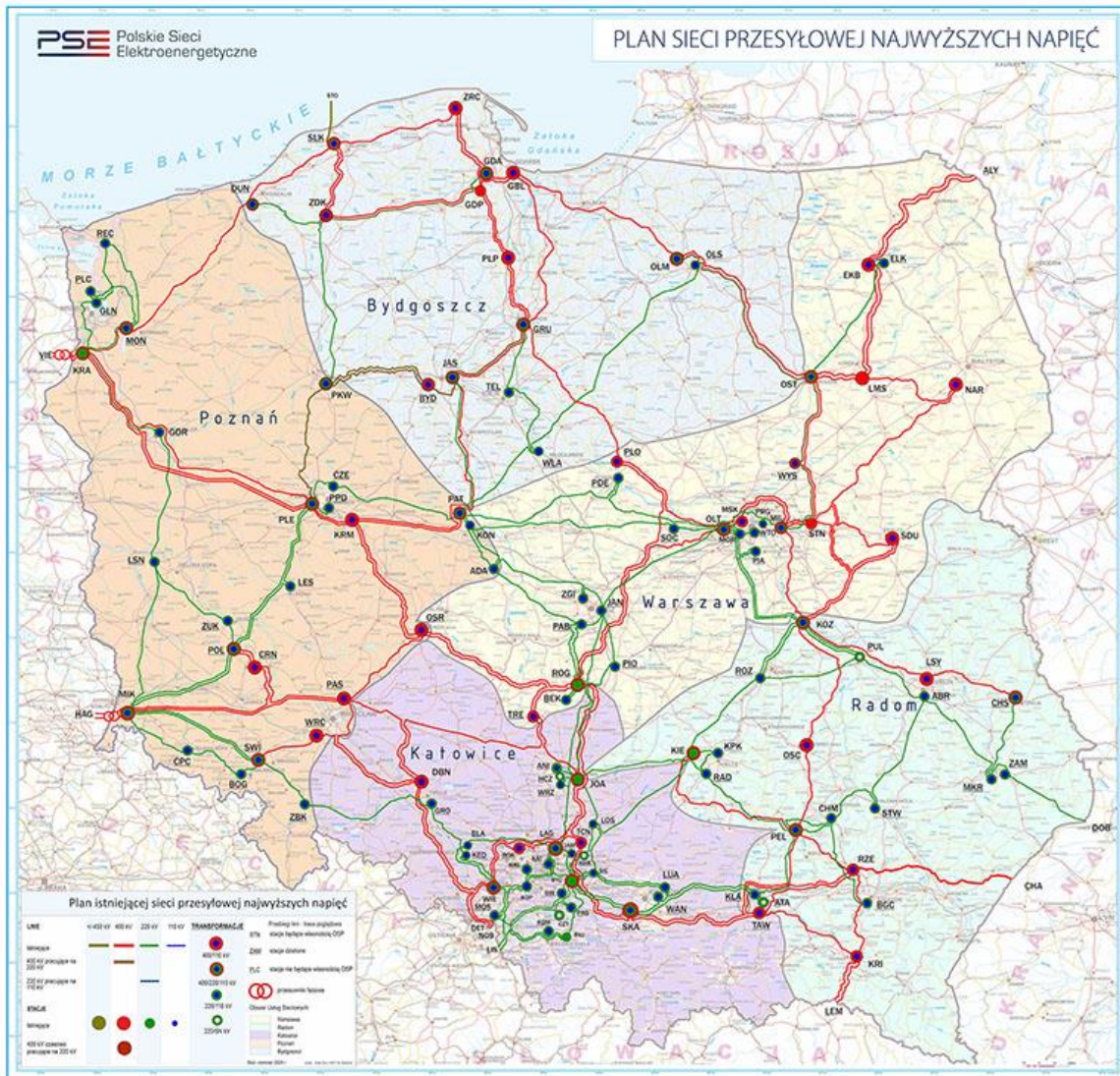
Rysunek 13 Schemat Krajowej Sieci Przesyłowej Źródło: PSE, www.pse.pl , data dostępu: 22.03.2024
